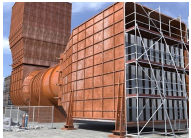
Abb. 153 Schalldämpferkulissen
