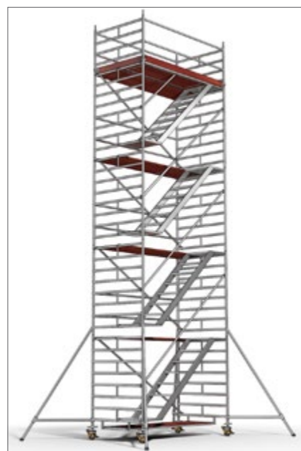
Abb. 56 Fahrbare Arbeitsbühne mit Treppenaufstieg und Abstützungen
