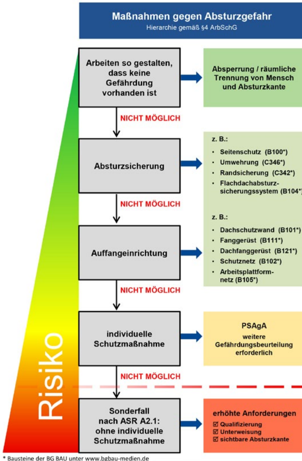
Abb. 9 Maßnahmen gegen Absturzgefahr
