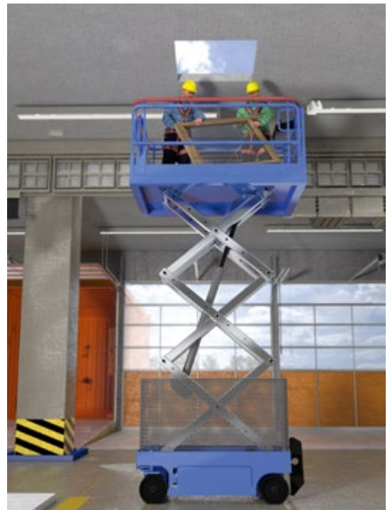
Abb. 62 Scherenbühne
