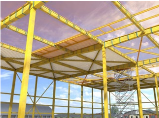
Abb. 125 Schutznetze
