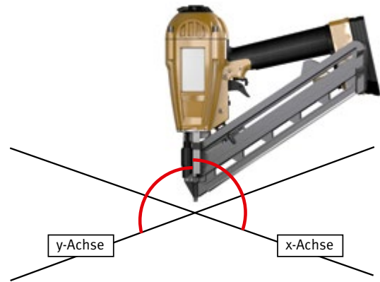
Abb. 147 Positionierung des Schussapparates
