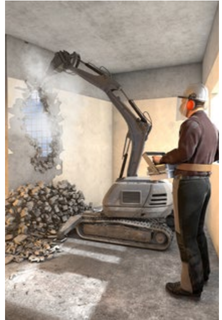
Abb. 88 ferngesteuertes Abbruchgerät
