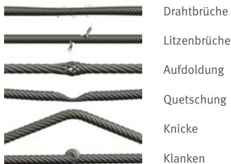
Abb. 81 Beispiele für Ablegekriterien von Drahtseilen
