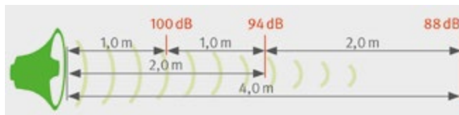
Abb. 29 Schallpegelabnahme durch Entfernung
